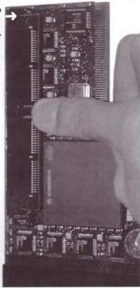
Pin1 / Aussparung
