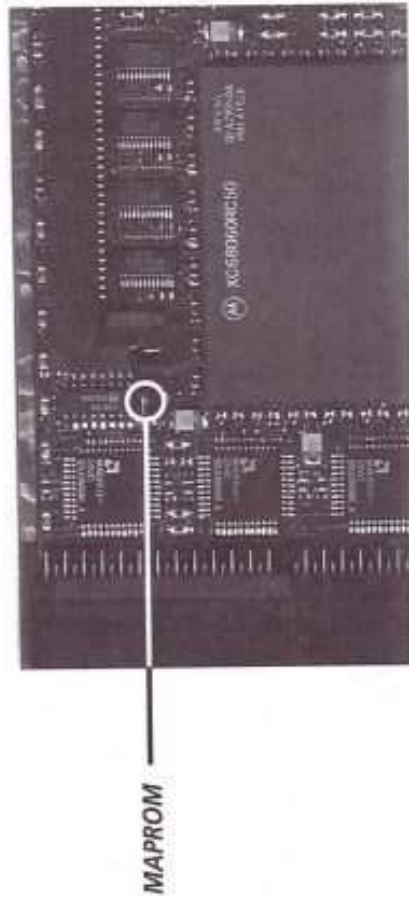
Bild 4 – MAPROM Jumper
