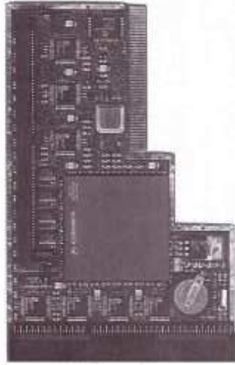
Bild 1 – Das BLIZZARD 1260 Turbo Board
